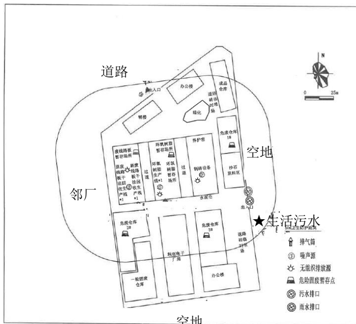
附图4.1-3 厂区平面布置图
